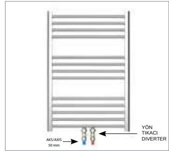
3- ORTADAN GİRİŞ - ÇIKIŞLI BAĞLANTI 3 - MIDDLE INLET/OUTLET CONNECTION
